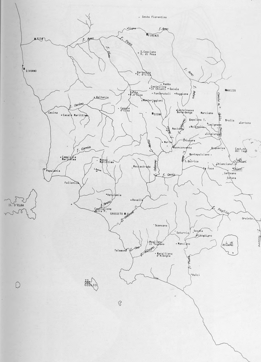
1. Il bacino idrografico dell'Ombrone e le altre vie d'acqua dell'Etruria settentrionale.
