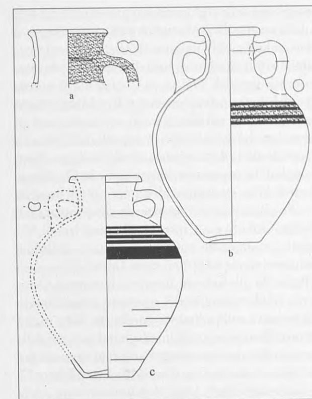
Fig. 4. Anfora tipo Cruz del Negro: a, dall'abitato di Sulcis (Bartoloni 1990, fig. 7, 125) (scala 1:4); b, da Monte Sirai (P. Bartoloni, La necropoli di Monte Sirai - I , Roma 2000, fig. 30, 72); c, da Ibiza (Gómez Bellard et al. 1990, fig. 11, 28) (scala 1:6).
