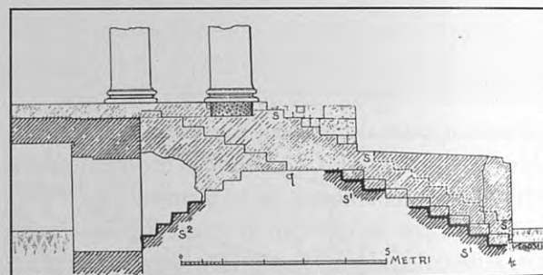
Fig. 20. Tempio di Giove: sezione della scalinata e del podio, con le due fasi di costruzione (da Maiuri 1973).
