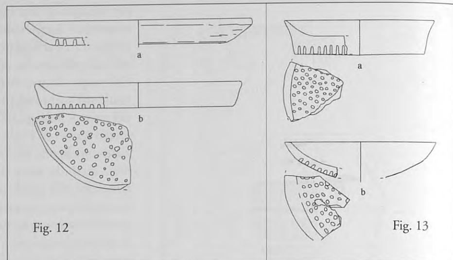
Fig. 12. Piatto con perforazioni sulla superficie esterna: a, da Cartagine (Mansel 1999, tav. 5, 46); b, da Morro de Mezquitilla (Schubart 1983, fig. 12, b) (scala 1:4). Fig. 13. Piatto con perforazioni sulla superficie esterna: a-b, da Morro de Mezquitilla (Schubart 1983, fig. 12, d, f) (scala 1:6).
